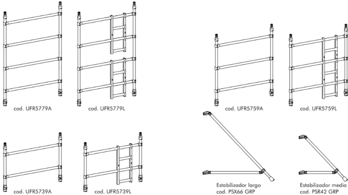
Bastidores de estension anchos
