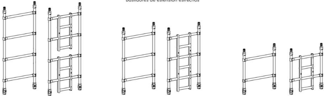
Bastidores de estension estrechos
